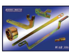
Blokada rozrządu 2,0 / 2,1 / 2,2 CDI Mercedes
