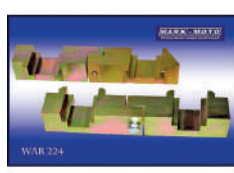
Blokada wałków rozrządu BMW benzyna M60 / M62
